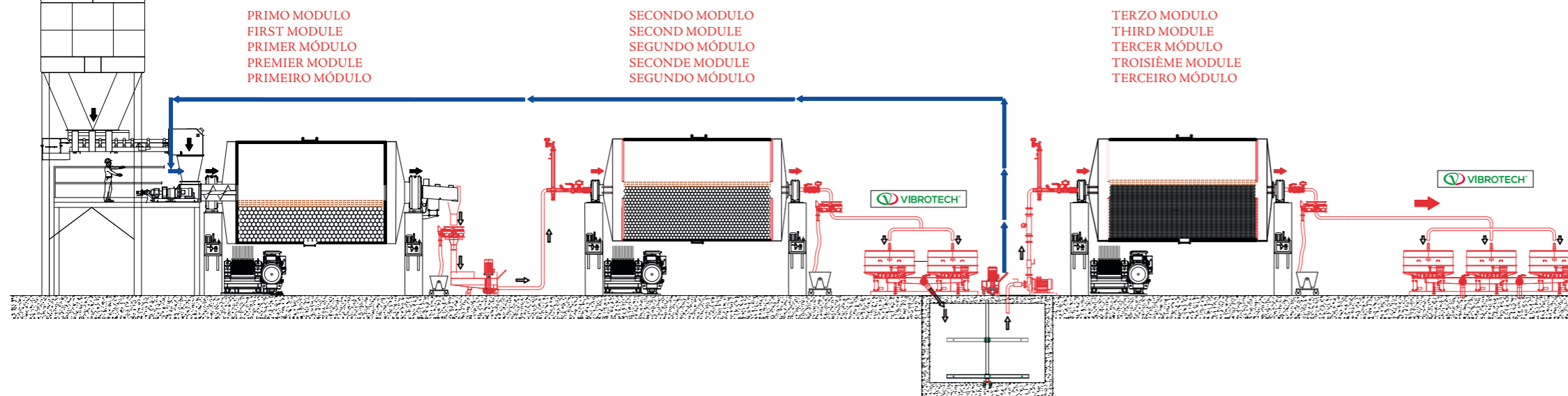
SCHEMA MULINI MODULARI TIPO CERTECH. DIAGRAM OF MODULAR MILLS TYPE CERTECH ESQUEMA MOLINOS MODULARES TIPO CERTECH. SCHEMA BROYEUR MODULAIRES CERTECH ESQUEMA DE MOINHOS MODULARES TIPO CERTECH
